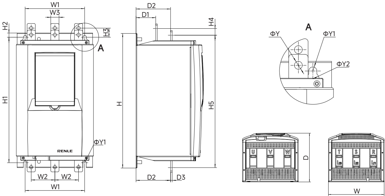
外形及安装尺寸表：（请对照上图进行参数查询）
