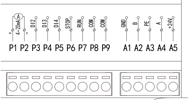
外控端子示意图
