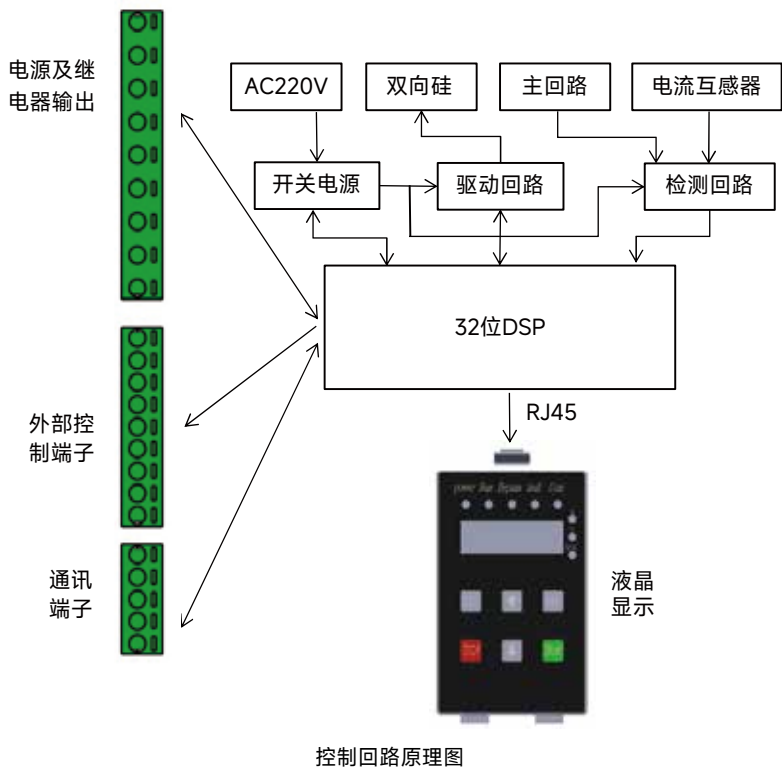
控制回路原理图
