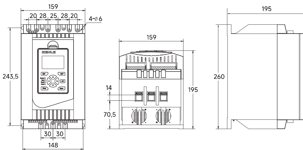
① M0 产品外形及安装尺寸
